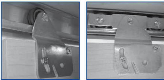
RILAJ2, RILAJ3, RIALJ2 y RIALJ3 Para deslizar los sistemas de carretillas CCLOS y CCLOD.
